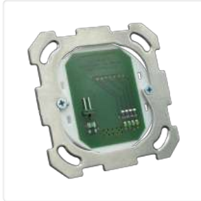
X-IC-29-0001 IC T4-PLUG-IN Modul
